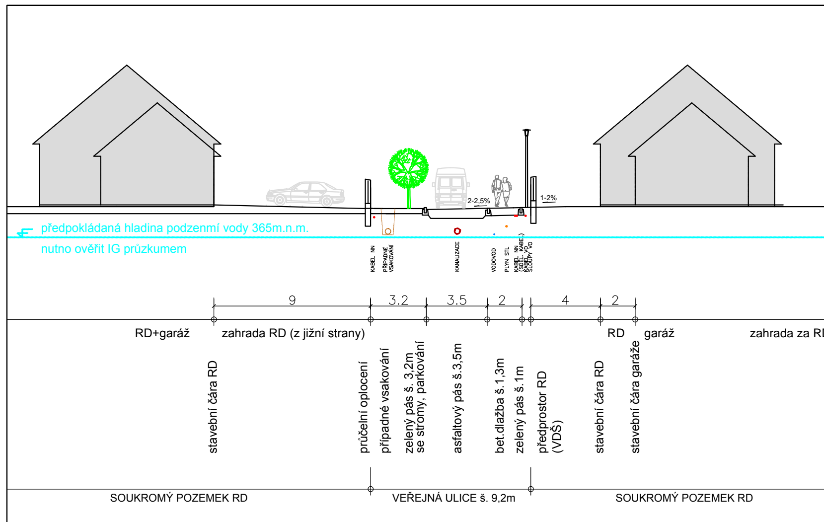
ŘEZ A-A - schematický příčný řez ulicí spojovací
